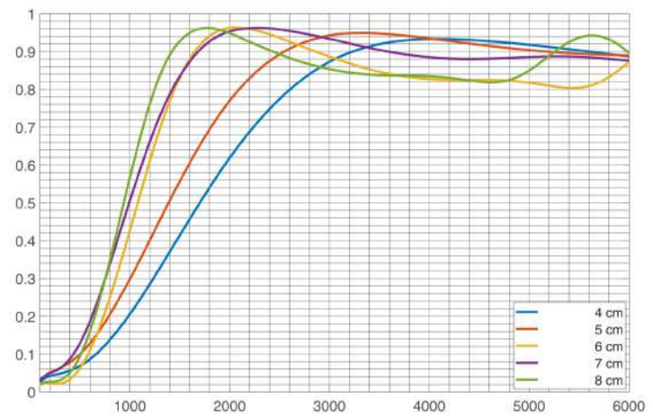
Simulation des Schallabsorptionskoeffizienten mit Thomasson-Korrektur
